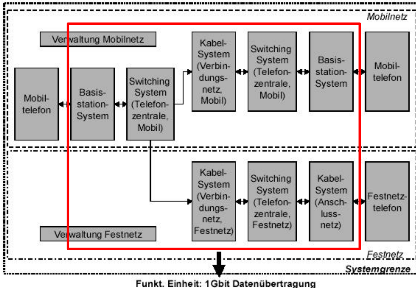
Fig. 2.1: Betrachtete Elemente des Mobilfunksystems UMTS. 1 Gbit = 1'000'000 kbit. Die Studie betrachtet das Mobilnetz und das Festnetz, das für eine Datenübertragung von Mobil- zu Festnetz nötig ist.
